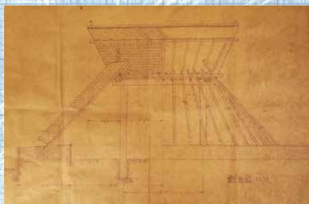
関野克「登呂復元竪穴家屋設計図（断面図）」
